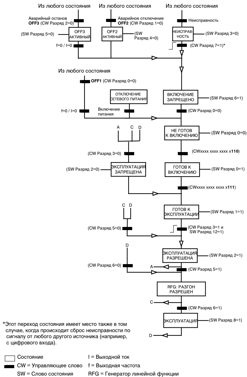
Рис. 69. Конечный автомат для оценки сигналов пуска и останова.
