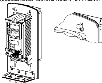
Рис. 7 Крепление преобразователей частоты типа IP 54 / NEMA12.
