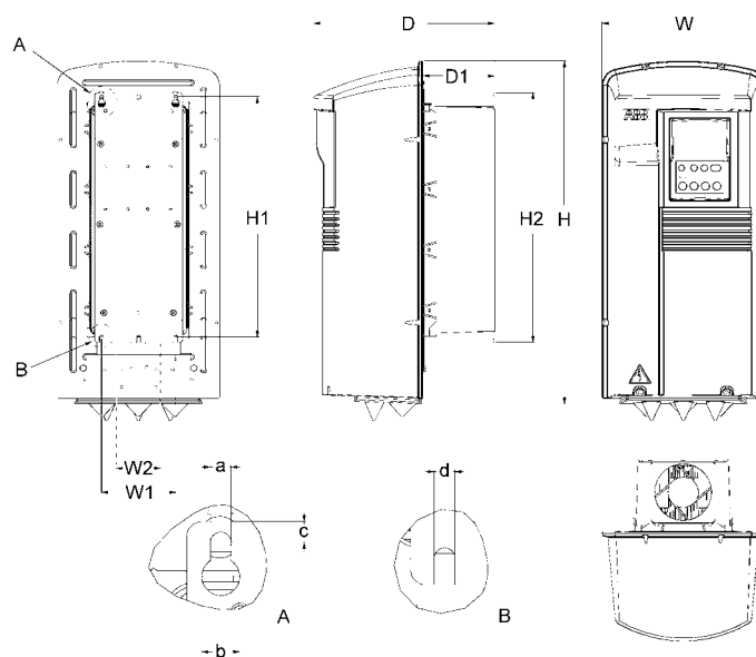
Рис. 3 Корпуса IP 54/NEMA12
