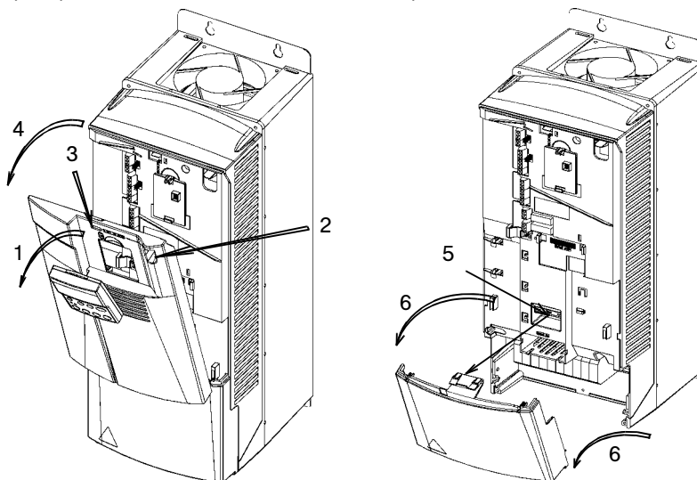
Рис. 9 Открытие преобразователей частоты с рамой размера R3 и R4 типа IP 21 / NEMA1.
