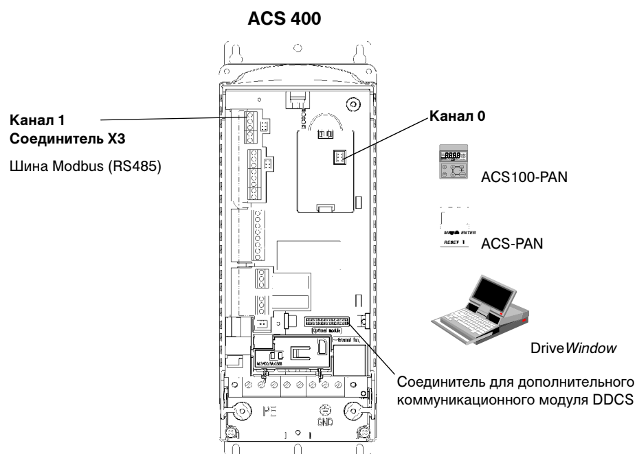
Рис. 66. Изображение средств стандартной связи по последовательному каналу преобразователя ACS 400.
