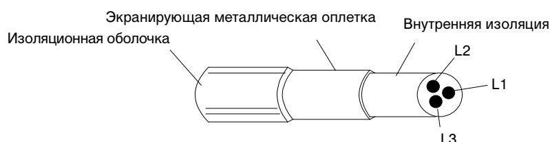
Рисунок 79 .Эффективное экранирование кабеля электродвигателя (например, кабели Ciflex-Servo-FD 780 CP, Lappkabel или MCCMK, NK).
