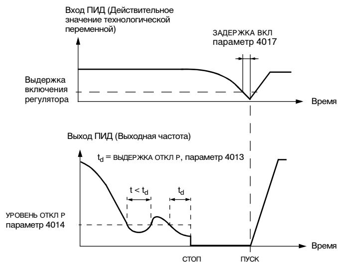
Рис. 56. Действие функции отключения регулятора.
