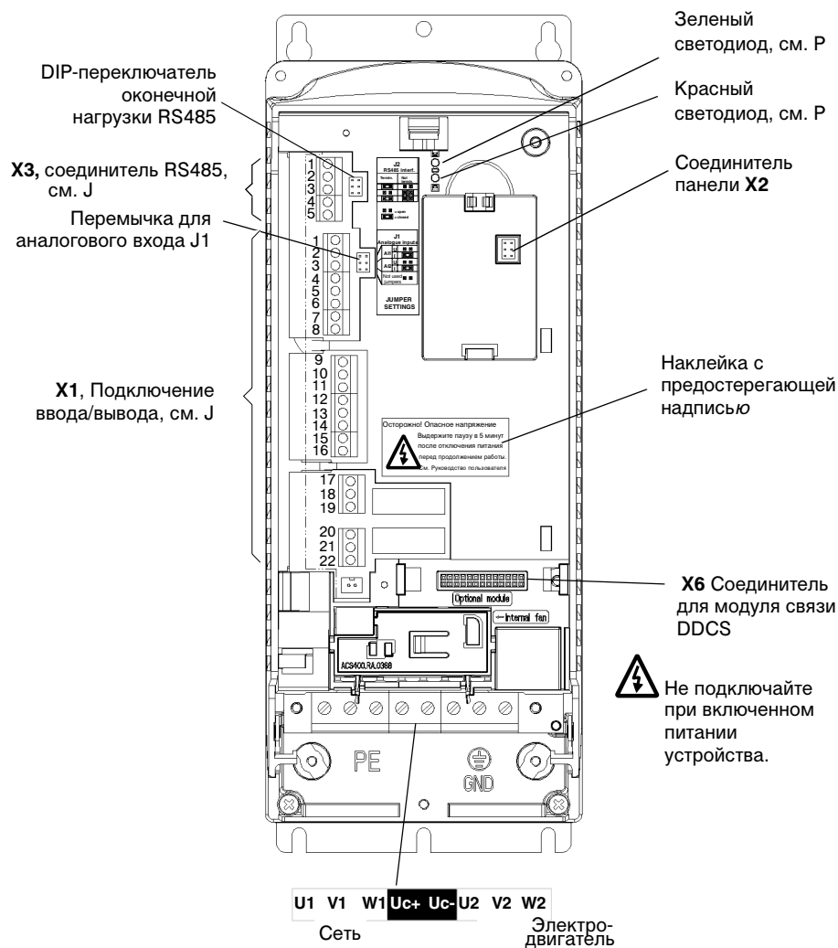
Рис. 11 Контактные колодки.
