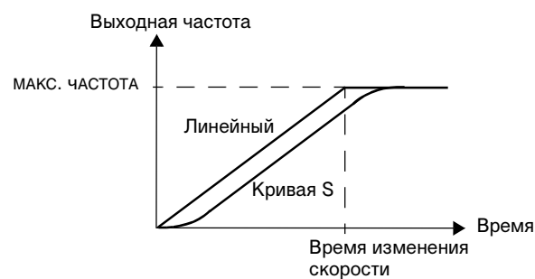
Рис. 42. Определение времени участка ускорения/замедления.
