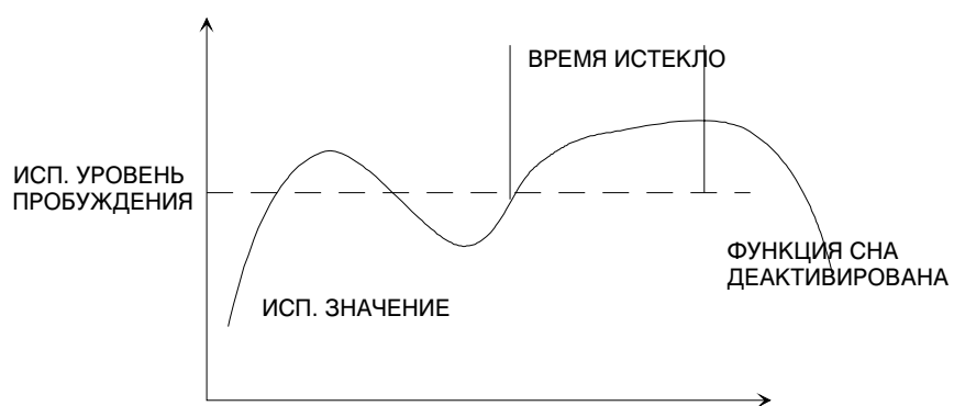
Рис. 60. Использование уровня пробуждения с инвертированным значением ошибки.
