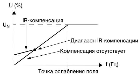
Рис. 44. Принцип действия IR-компенсации
