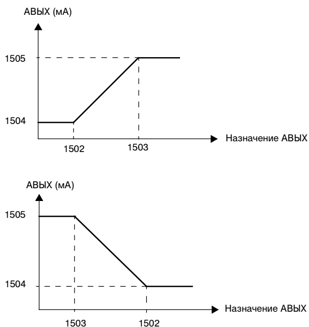
Рис. 41. Масштабирование аналогового выхода.
