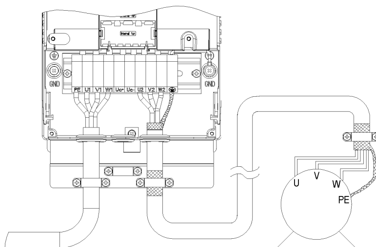
Рис. 20 Подключение кабеля электродвигателя для рам размеров R3 и R4 (IP 21 / NEMA1).
