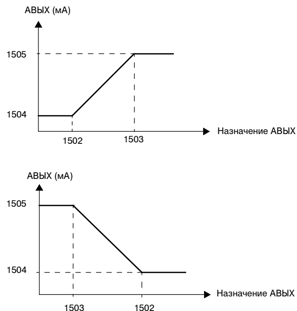
Рис.9 Масштабирование аналогового выхода.
