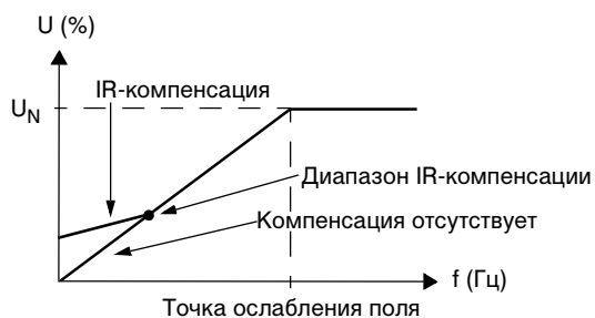
Рис.12 Принцип действия IR-компенсации
