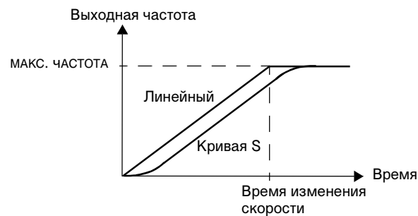
Рис. 10 Определение времени участка ускорения/замедления.
