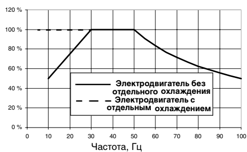
Понижение в зависимости от выходной частоты (электродвигатели ABB M3VA/AA, M2VA/AA, M3VRF/S and M3ARF/S)
