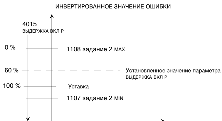
Рис.25 Пример смещения установленного значения уровня деактивации функции отключения; параметр 4015 WAKE-UP LEVEL равен 60 %, ПИД-управление с инверсией.
