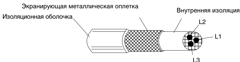
Рис. 34 Эффективное экранирование кабеля электродвигателя (например, кабели Ciflex-Servo-FD 780 CP, Lappkabel или MCCMK, NK).
