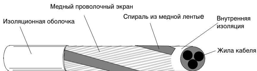
Рис. 32 Минимальные требования в отношении экранирования кабеля электродвигателя (например, кабели MCMK, NK)
