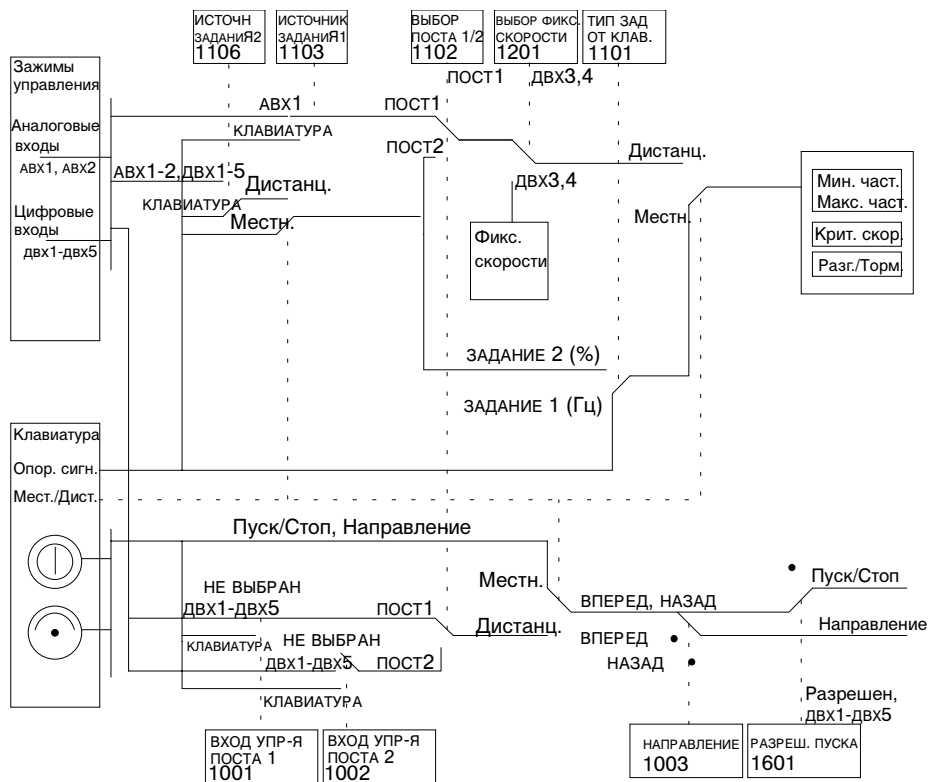
Рис. 30 Схема прохождения сигналов управления для макросов стандарта ABB, изменения направления и предварительного намагничивания.
