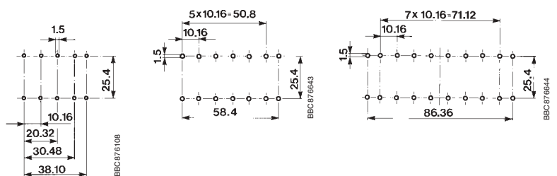
4-полюсный аппарат
