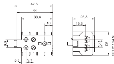
Блок вспомогательных контактов САФ 6 с винтовыми зажимами
