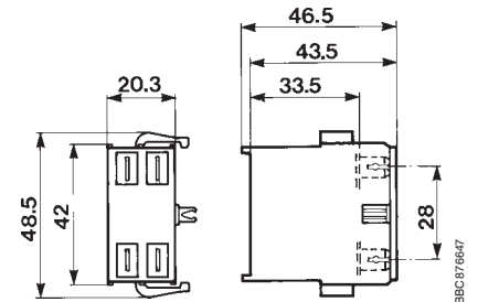
Блок вспомогательных СА 6- F со штырьковыми соединениями
