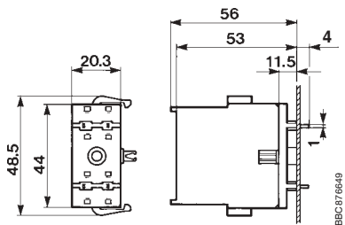
Блок вспомогательных контактов СА 6 + LB 6- СА
