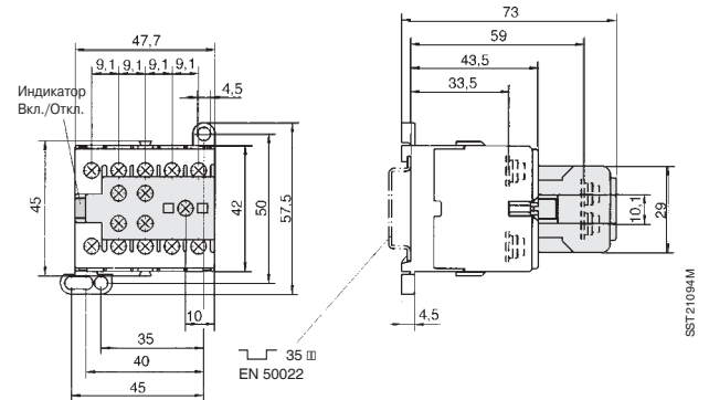
В 6, В 7, ВС 6, ВС 7, К 6, КС 6 + блок вспомогательных контактов фронтальной установки САФ 6
