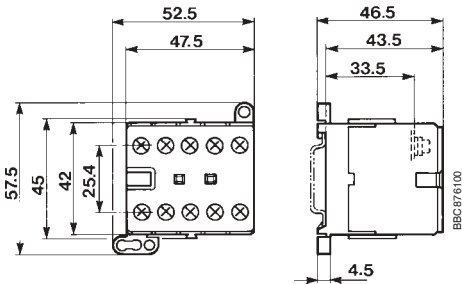
В 6, В 7, ВС 6, ВС 7, К 6, КС 6 с винтовыми зажимами
